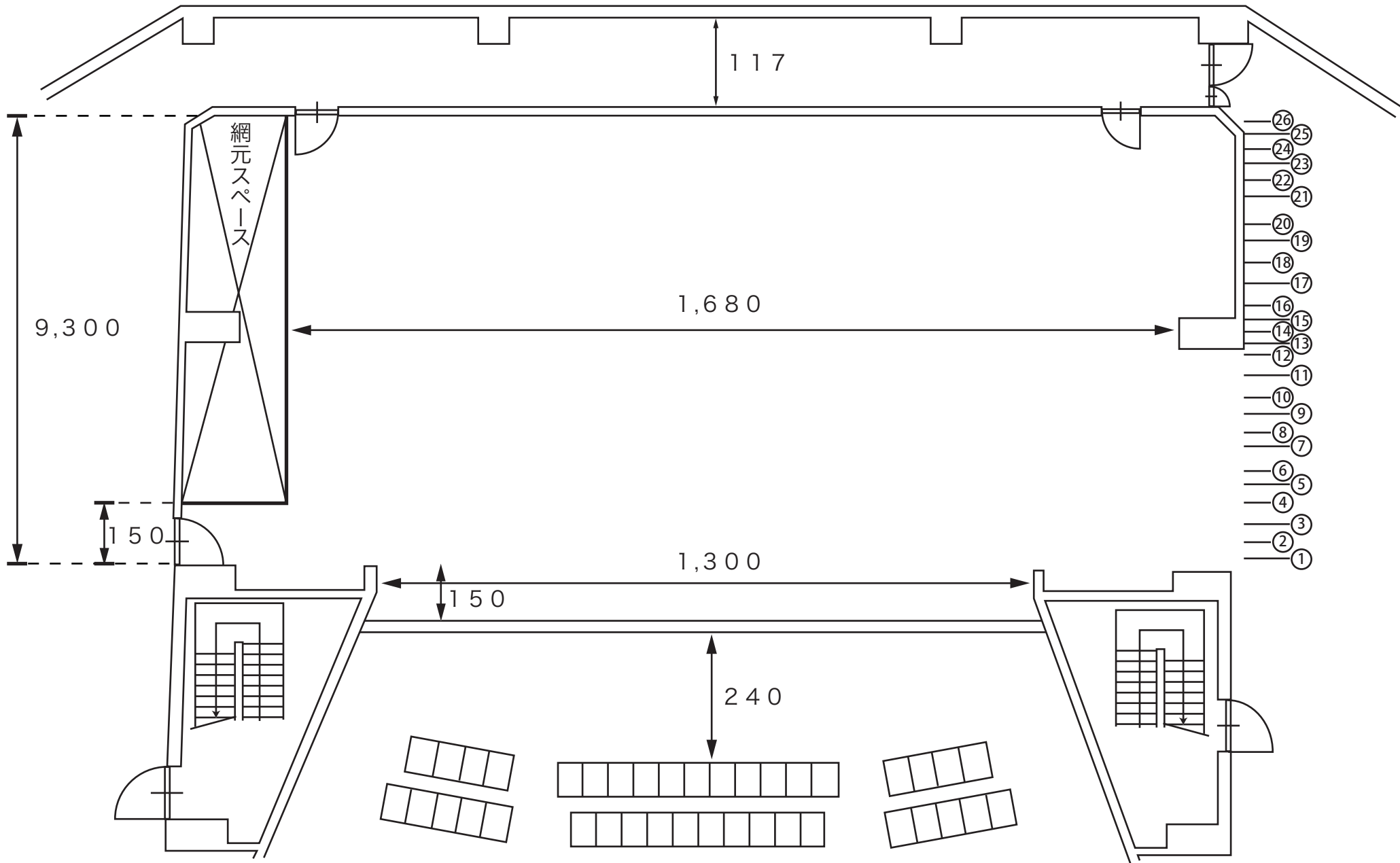
長岡市中之島文化センター 舞台 平面図 (単位 : cm)
